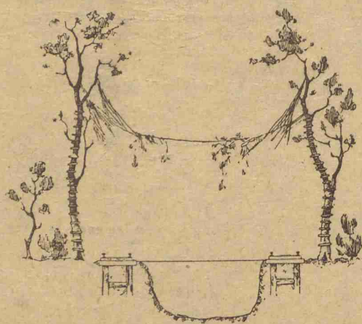
Corte transversal y altura de la plataforma del cañón número 3 de esta misma batería. De árbol a árbol pasa una red metálica que cubierta de hojas y maleza impedía completamente la visibilidad aérea de la pieza. Por los árboles suben unas pequeñas escaleras destinadas a la observación. El foso, de una profundidad de un tercio de la altura de la pieza, contribuía a emboscar perfectamente este emplazamiento artillero.
