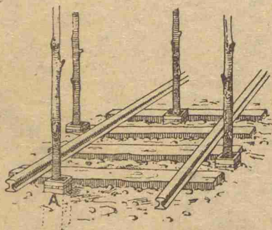
Disposición de los cajoncillos destinados a soportar los árboles de quita y pon.
