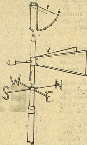
Anemómetro-Veleta de Wild
