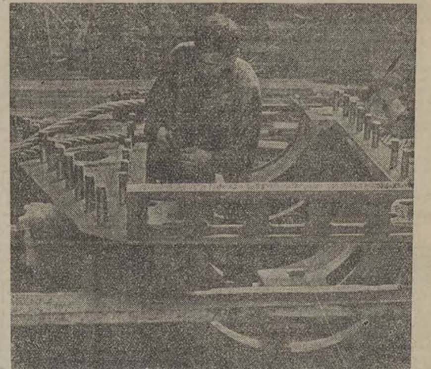
El cilindro de una turbina de 100.000 caballos de fuerza de la fábrica Stalin, de Leningrado.
