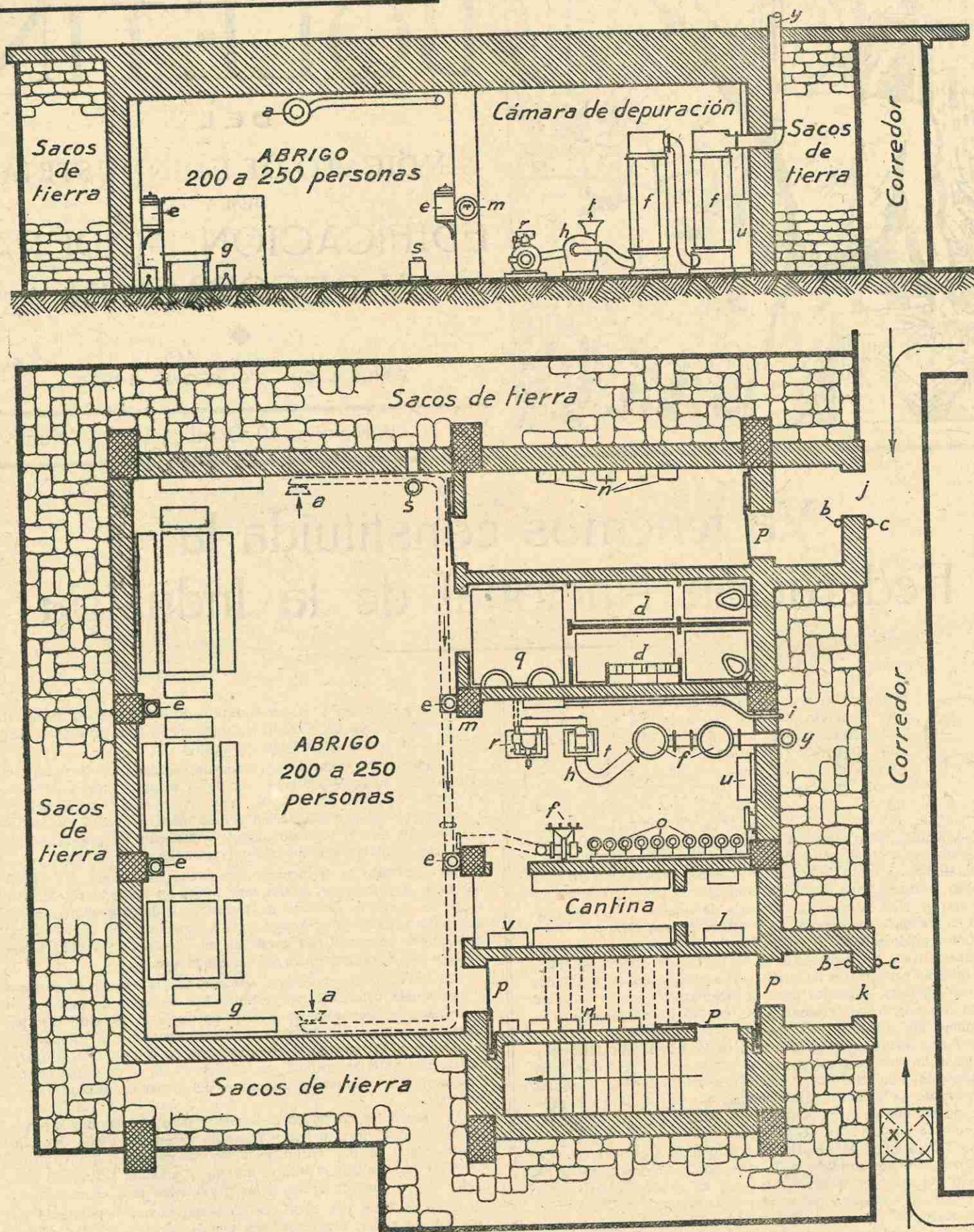
Figuras 1 y 2: Corte vertical y horizontal del refugio subterráneo.
