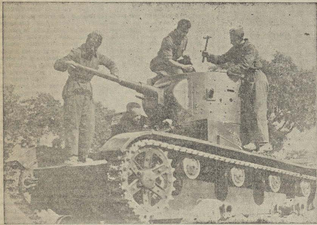
La avería sufrida en el tanque es inmediatamente reparada por los hábiles y valientes muchachos de los grupos tanquistas. (Foto Yubero y Benítez.)
