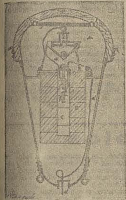
Torpedo electro-automático. A. Flotador B. Carga explosiva. C. Carga de fulminante. P. Puerta de carga; a', conductor; b', bola de metal; ff', fulminantes. Sección interior
