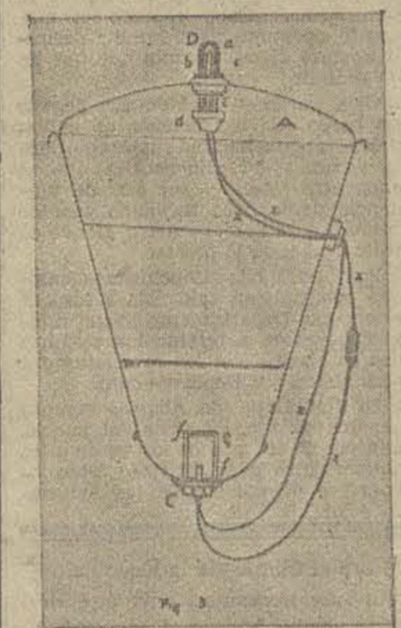
Torpedo electro-mecánico. (Sec. interior)
