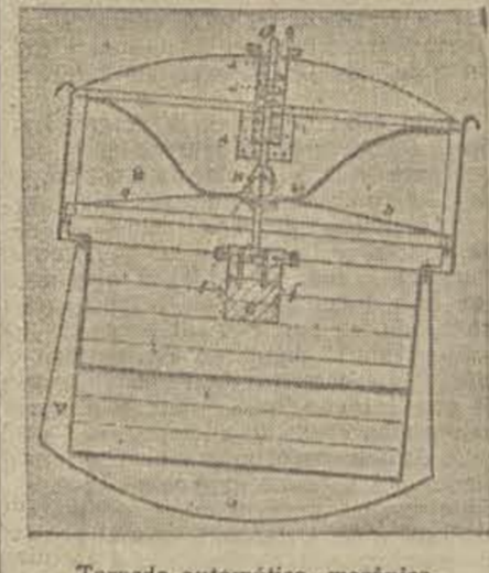
Torpedo automático-mecánico Sección interior
